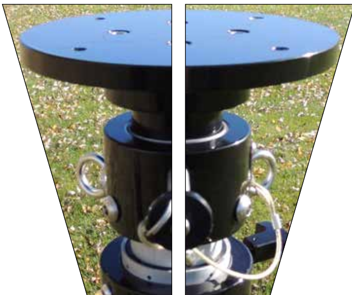
Abnehmbarer Nutzlastadapter
