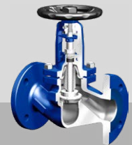
Faltenbalg-Ventil FABIA® Plus
